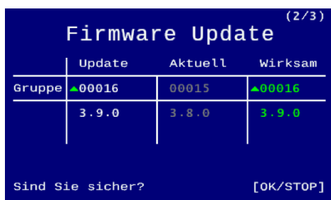
Abbildung 51: Informationen über die Update-Datei (2/3)
